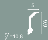
C321 | C321F 200 x 9,9 x 5 cm Purotouch®
