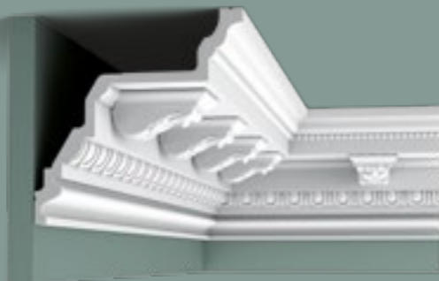
1 C307 + C307A 2 C307A: 7,5 x 4 x 9,4 Duropolymer® 19,5 9,4 4 5,6 ∇ = 26,9
