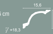
C217 | C217F 200 x 15,6 x 10,3 cm Purotouch®
