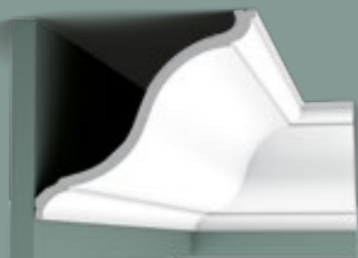
C335 200 x 20,2 x 22,2 cm Purotouch® Designed by Xavier Donck 22,2 20,2 ∇ = 29,3
